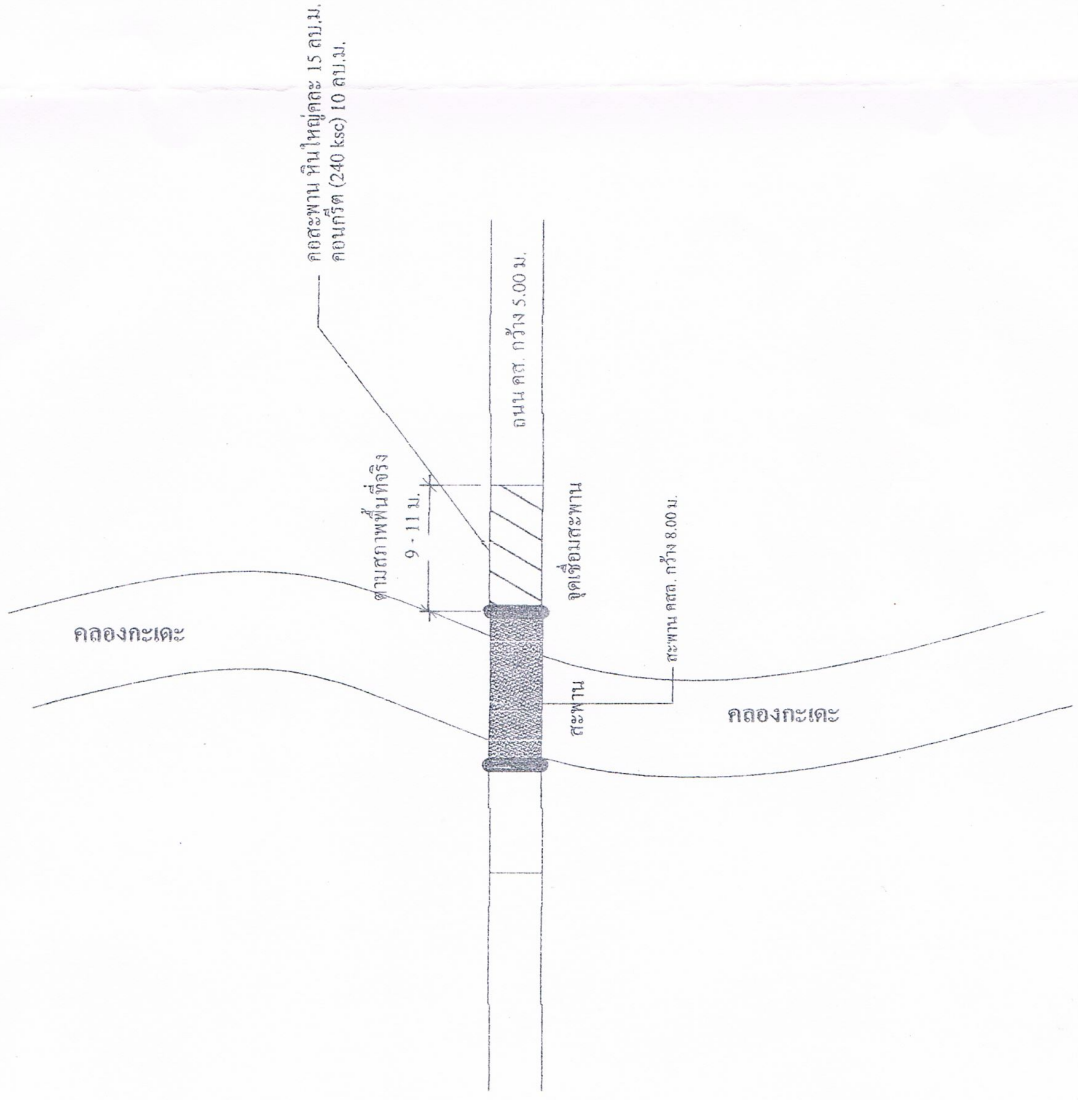
แบบขยายจุดเชื่อมสะพาน A
